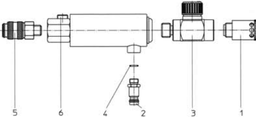
SATA air warmer, Atemluftwärmer
