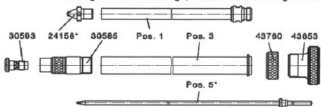
Tellerinnenmischverlängerung/Plate-shaped internal mixing extension/Rallonge, buse-assiette melangeur int.
